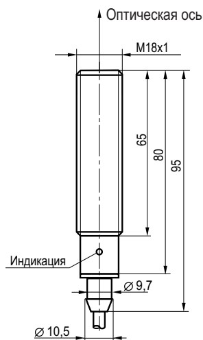
Габаритный чертеж
