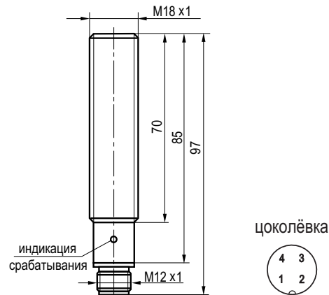
Габаритный чертеж.
