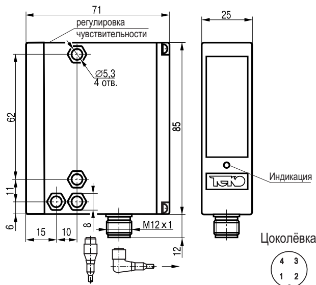
Габаритный чертеж
