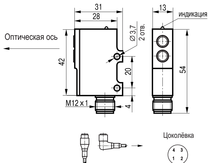
Габаритный чертеж
