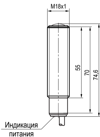
Габаритный чертеж
