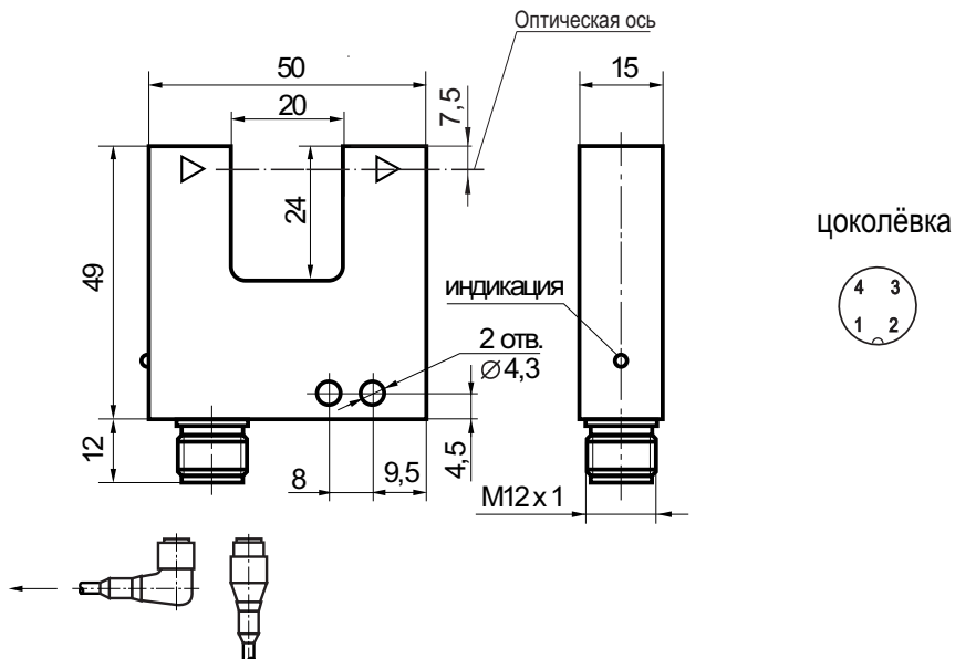
Габаритный чертеж
