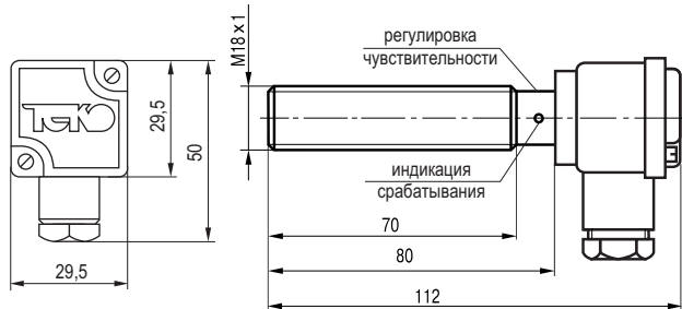
Габаритный чертеж.
