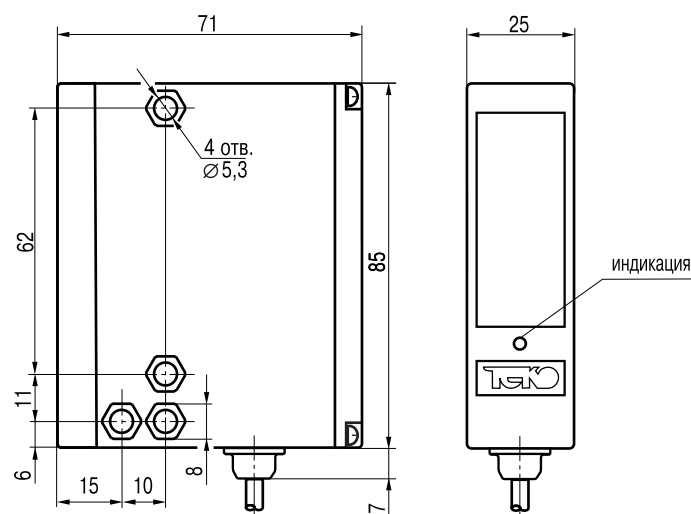
Габаритный чертеж
