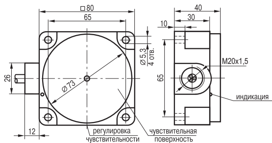
Габаритный чертеж
