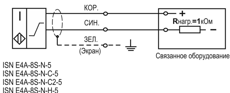
Схема подключения к оборудованию
