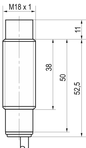
Габаритный чертеж
